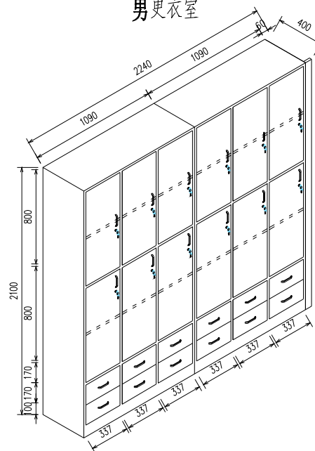
女更衣柜 规格: 2240L*400W*2100Hmm 数量: 1组 材质: 柜体: 1.0mm厚电解板加工, 环氧树脂喷涂 (半光白9003)
