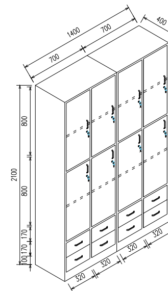
女更衣柜 规格: 1400L*400W*2100Hmm 数量: 1组 材质: 柜体: 1.0mm厚电解板加工, 环氧树脂喷涂 (半光白9003)
